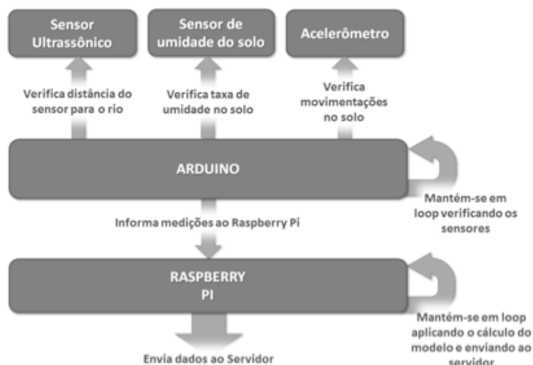
Figura 1. Funcionamento do Módulo de Sensores
